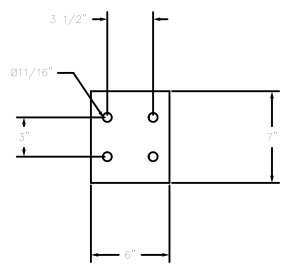
DETAIL A-A (TYP)
