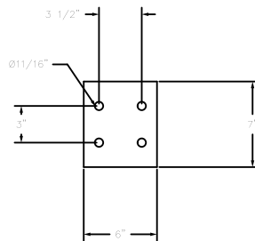
DETAIL A-A (TYP)
