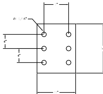
DETAIL A-A (TYP)
