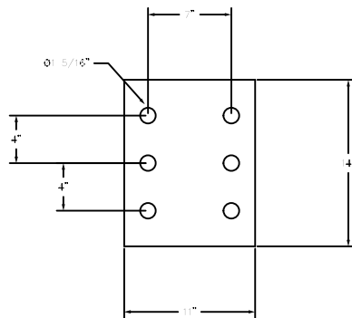
DETAIL A-A (TYP)
