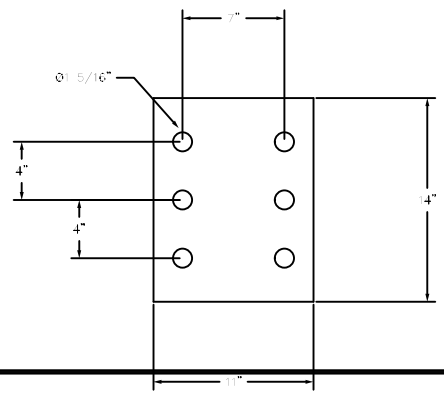
DETAIL A-A (TYP)
