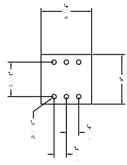
DETAIL A-A (TYP)
