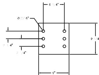
DETAIL A-A (TYP)
