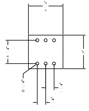
DETAIL A-A (TYP)
