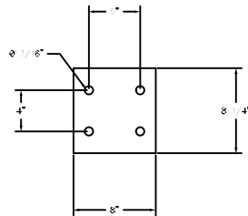
DETAIL A-A (TYP)
