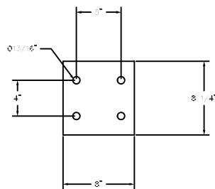
DETAIL A-A (TYP)
