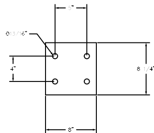
DETAIL A-A (TYP)
