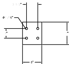
DETAIL A-A (TYP)
