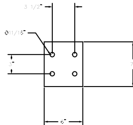
DETAIL A-A (TYP)
